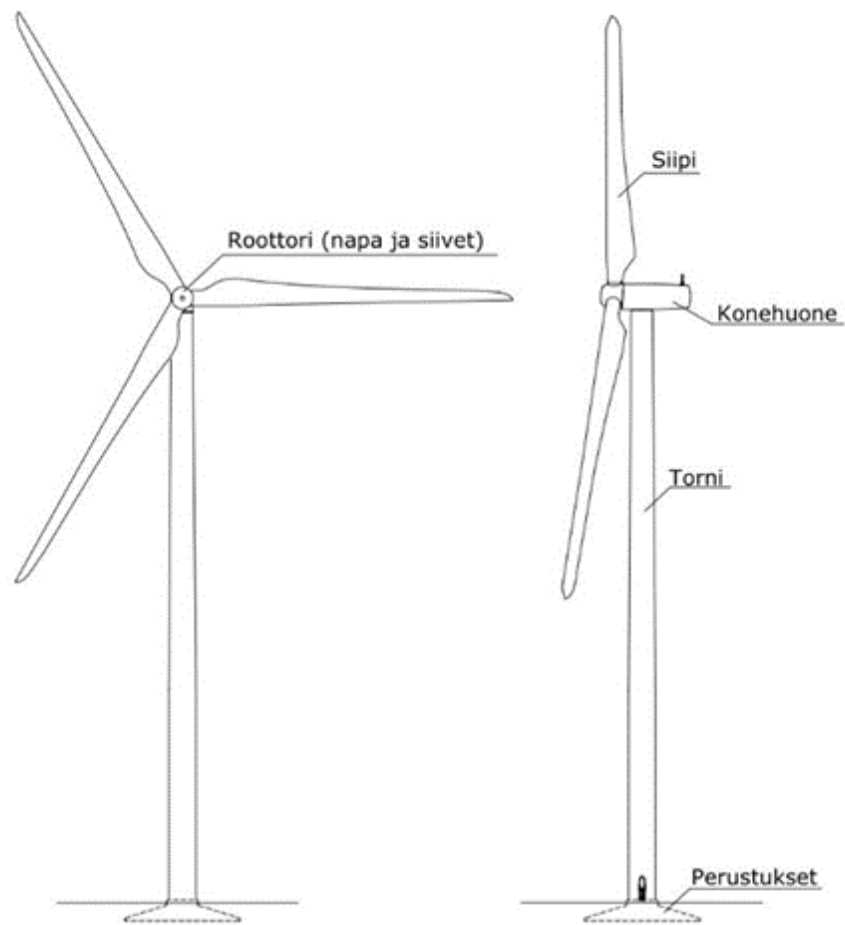
Kuva 3-1. Tuulivoimalan periaatekuva.
