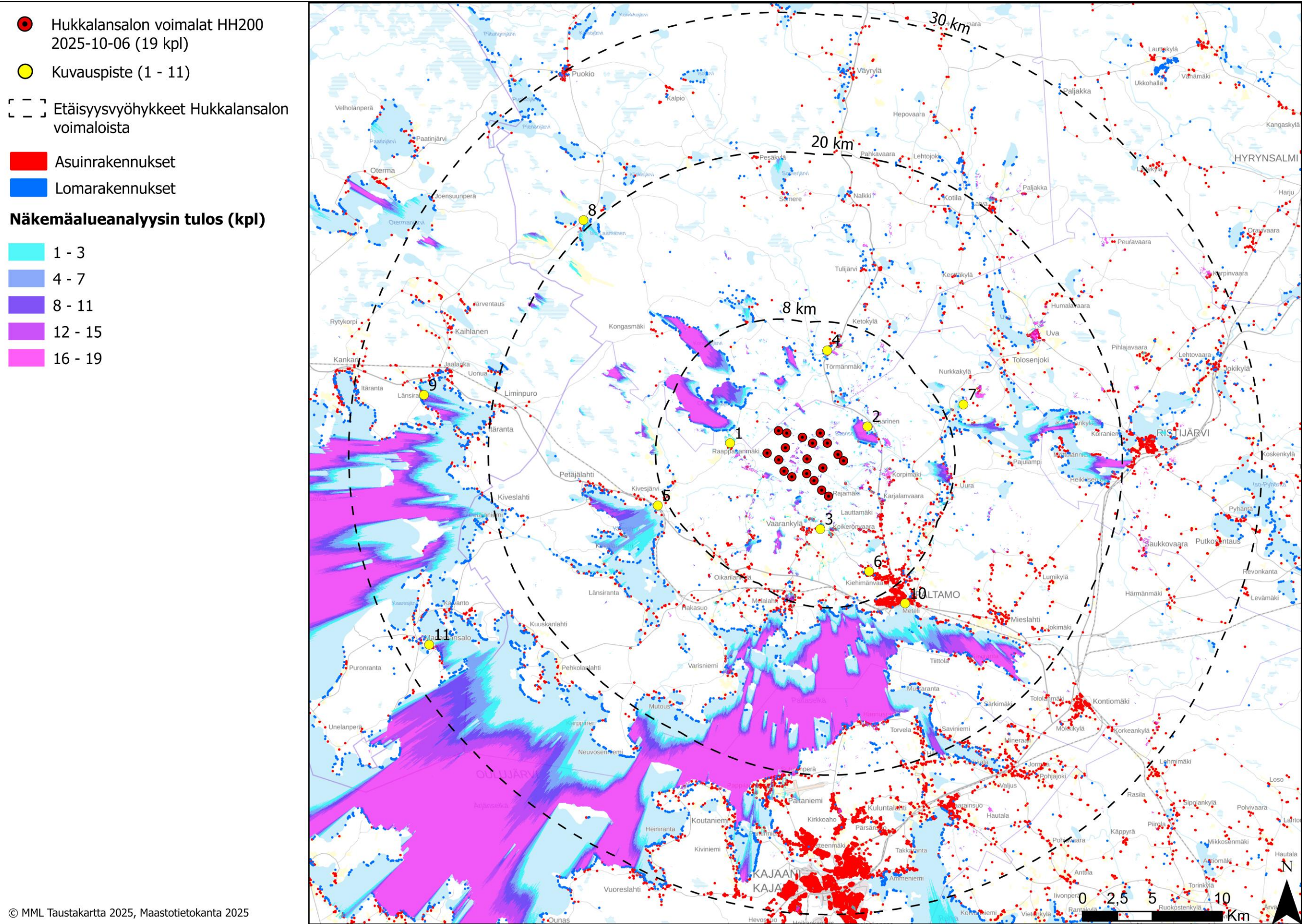
Kuva 1. Hukkalansalon tuulivoimahankkeen näkemäalueanalyysin laskentatulokset voimaloiden napakorkeudelle mallinnettuna.
