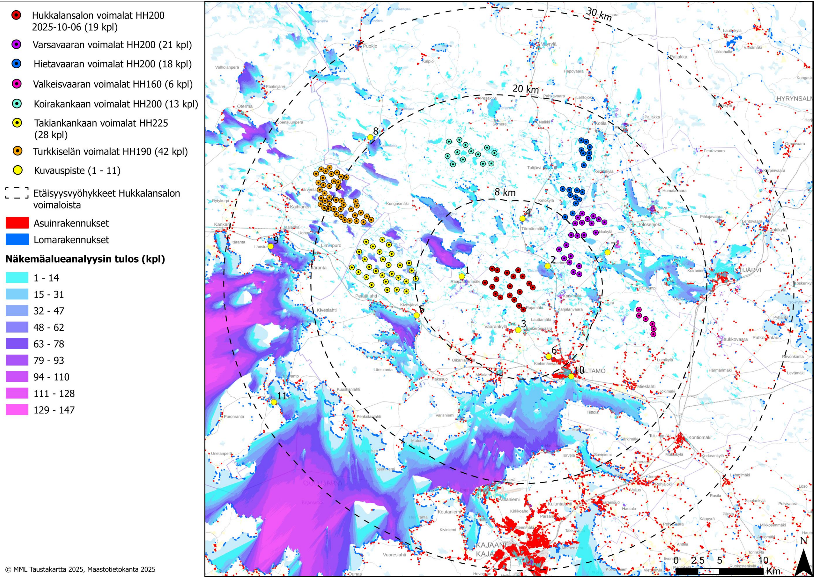
Kuva 24. Hukkalansalon tuulivoimahankkeen yhteisvaikutusten näkemäalueanalyysin laskentatulokset voimaloiden napakorkeuksilla mallinnettuna
