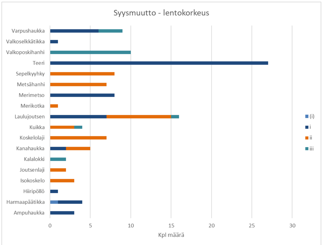
Kuva 33. Syysmuuton seurannassa havaittujen tuulivoiman kannalta huomionarvoisten muuttolintujen lukumäärät lajeittain eri lentokorkeuksissa. Ensimmäinen aste on 0–100 metriä, toinen 100–300 metriä ja kolmas yli 300 metriä. Näistä toisen asteen lennot ovat ns. riskilentoja.
