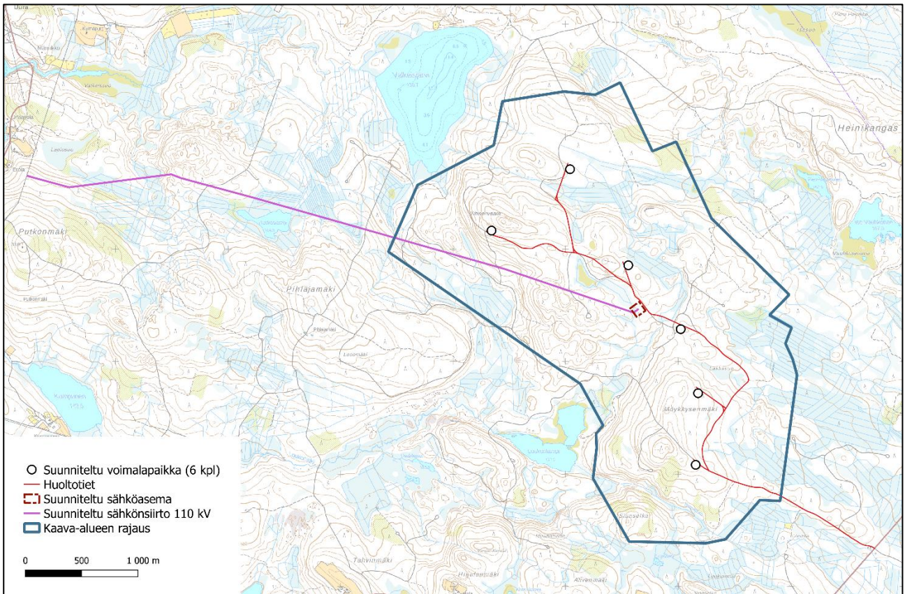
Kuva 2. Valkeisvaaran tuulivoimahankkeen alustava voimalasijoittelu, huoltotiet sekä suunniteltu ulkoinen sähkönsiirtoreitti. Sisäisen sähkönsiirron maakaapelireitit sijoittuvat huoltoteiden reunaan.
