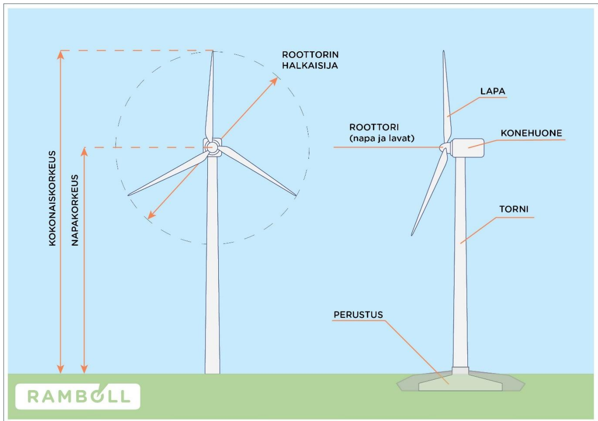
Kuva 3-1. Tuulivoimalan periaatekuva.
